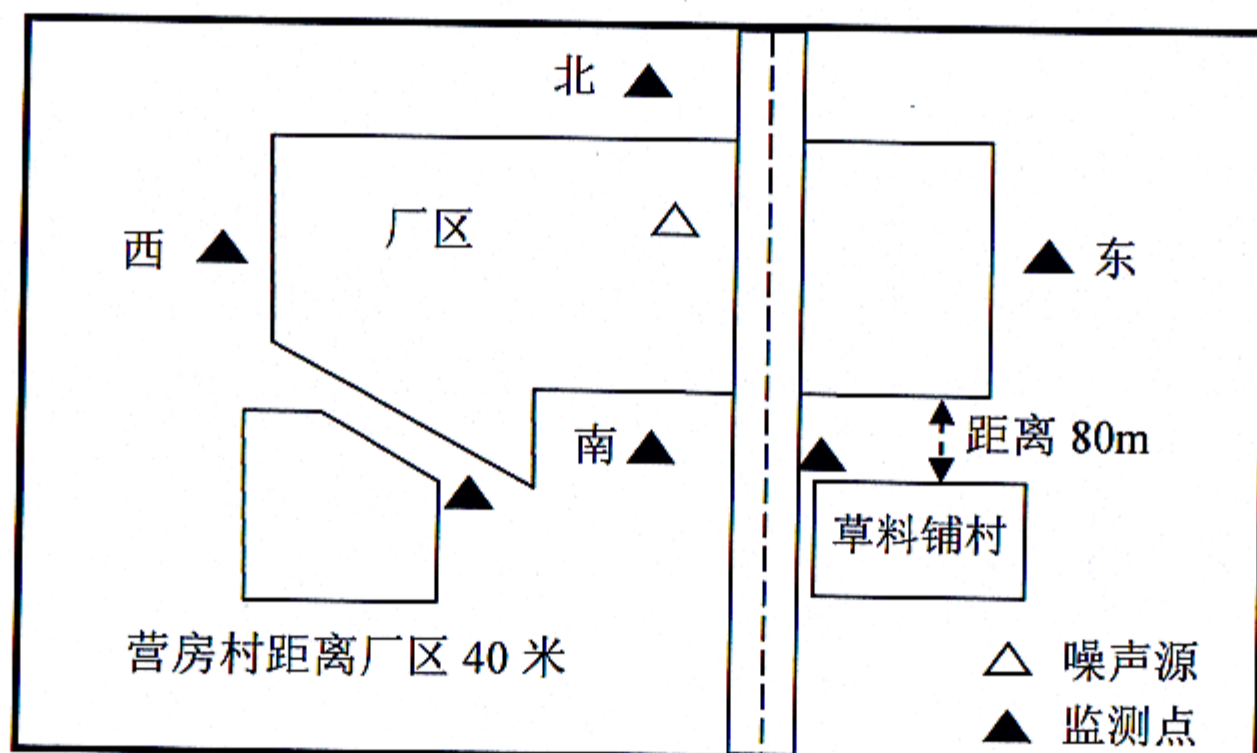
附图：噪声测试点示意图
