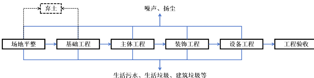
图 4-1 施工期工艺及污染工序
